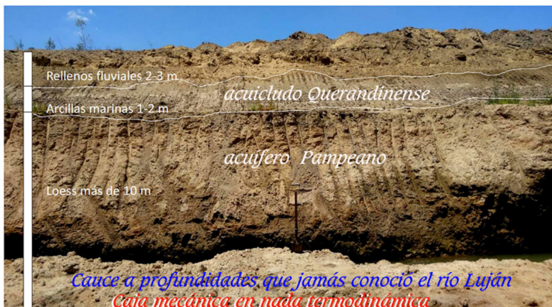
Figura 66: Perfil estratigráfico del área afectada por la obra de ampliación del canal Santa María.
